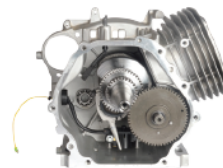
Motor de 4 tiempos
